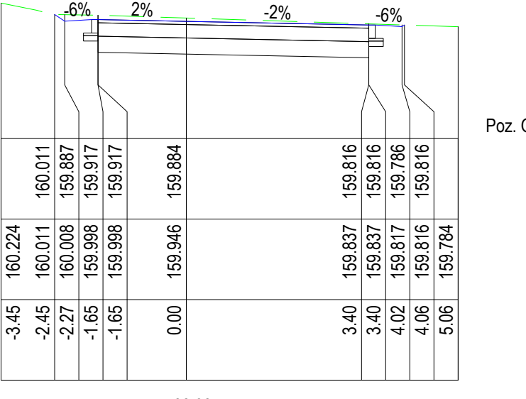
Poz. Odn. 157.7m Pik. 88.08 m Odcinek II
