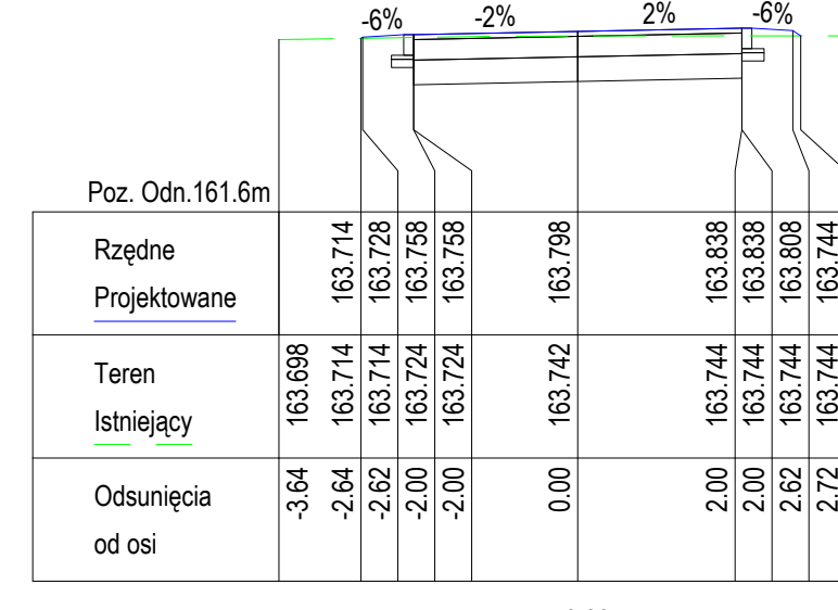
Poz. Odn. 161.6m Rzędne Projektowane Teren Istniejący Odsunięcia od osi
