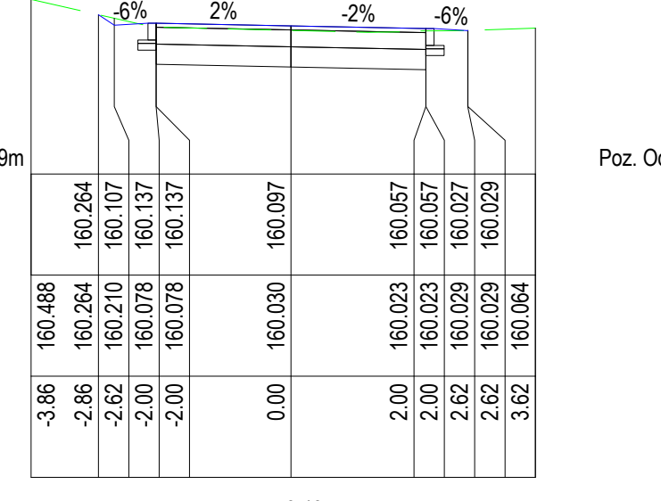
Poz. Odn. 157.9m Pik. 78.43 m Odcinek II
