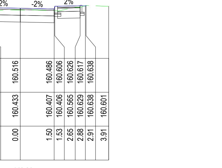
Poz. Odn. 158.3m Pik. 140.00 m Odcinek II
