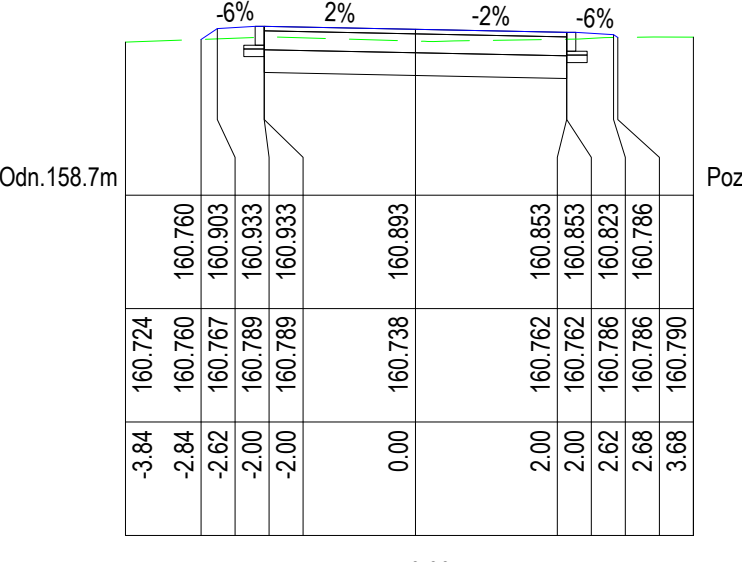
Poz. Odn. 158.7m Pik. 50.00 m Odcinek II
