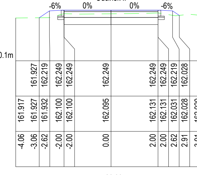
Poz. Odn. 160.1m Pik. 20.00 m Odcinek II
