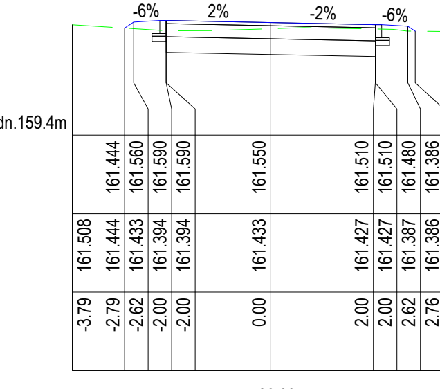
Poz. Odn. 159.4m Pik. 30.00 m Odcinek II
