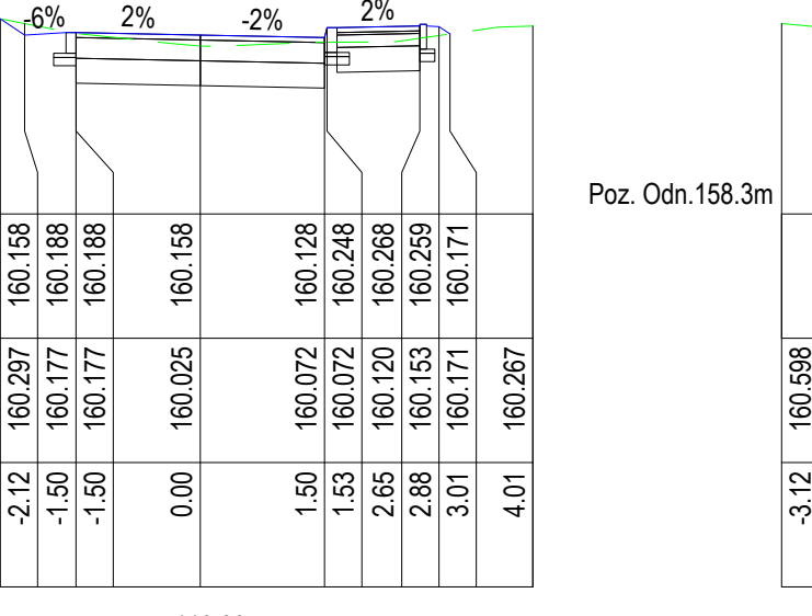
Poz. Odn. 158m Pik. 110.00 m Odcinek II
